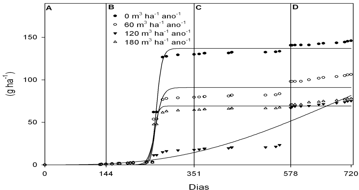
Figura 4.4. Perda acumulada de fósforo solúvel nas doses de 0, 60, 120 e 180 m 3 ha -1 ano -1 de dejetos líquido bovino aplicado em Latossolo Bruno sob plantio direto no período de 11/05/06 (dia 0) a 30/04/08 (dia 720), separando as estações do ano A, B, C e D, significando respectivamente Inverno 2006, Verão 2006/2007, Inverno de 2007 e Verão de 2007/2008. Total de 427 amostras analisadas.
