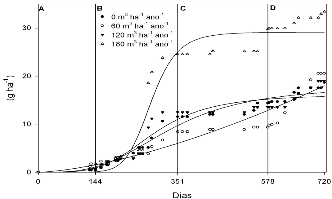
Figura 4.6. Perda acumulada de fósforo total nas doses de 0, 60, 120 e 180 m 3 ha -1 ano -1 de dejetos líquidos bovinos aplicados em Latossolo Bruno sob plantio direto no período de 11/05/06 (dia 0) a 30/04/08 (dia 720), separando as estações do ano A, B, C e D, significando respectivamente Inverno 2006, Verão 2006/2007, Inverno de 2007 e Verão de 2007/2008. Total de 192 amostras analisadas.
