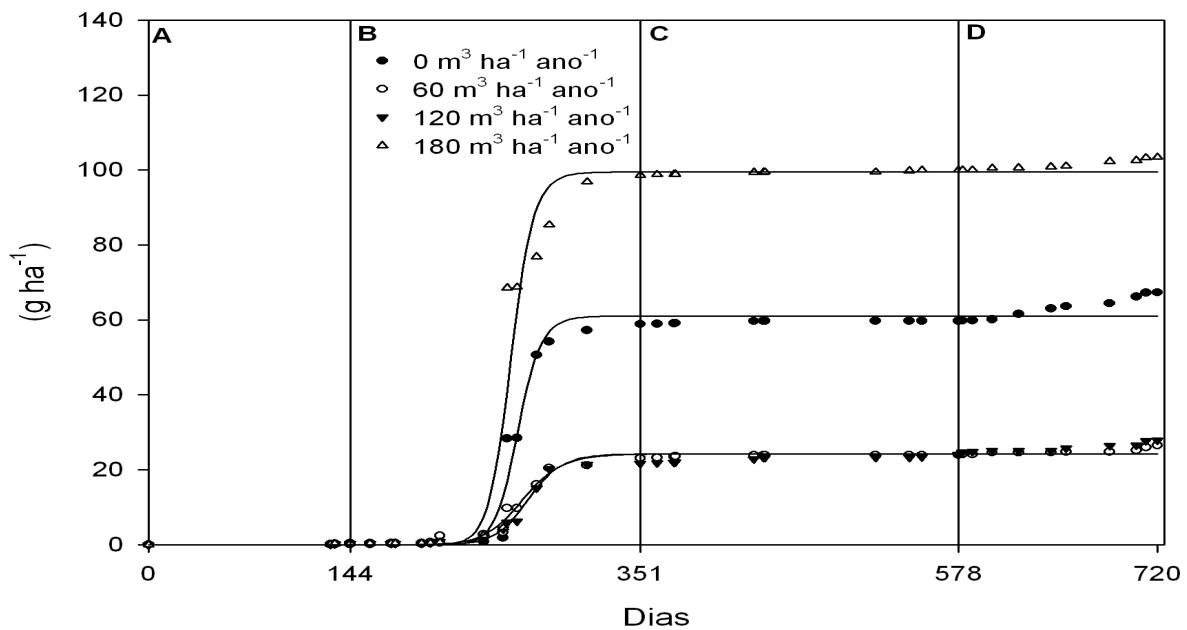
Figura 3.6. Perda acumulada de nitrato nas doses de 0 , 60 , 120 e 180 \text{ m}^3 \text{ ha}^{-1} \text{ ano}^{-1} de dejetos líquidos bovinos aplicados em Latossolo Bruno sob plantio direto no período de 11/05/06 (dia 0) a 30/04/08 (dia 720), separando as estações do ano A, B, C e D, significando respectivamente Inverno 2006, Verão 2006/2007, Inverno de 2007 e Verão de 2007/2008.
