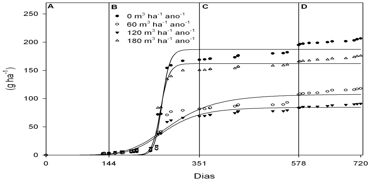
Figura 3.5. Perda acumulada de amônio nas doses de 0 , 60 , 120 e 180 \text{ m}^3 \text{ ha}^{-1} \text{ ano}^{-1} de dejetos líquidos bovinos aplicados em Latossolo Bruno sob plantio direto no período de 11/05/06 (dia 0) a 30/04/08 (dia 720), separando as estações do ano A, B, C e D, significando respectivamente Inverno 2006, Verão 2006/2007, Inverno de 2007 e Verão de 2007/2008.
