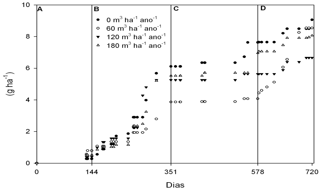
Figura 4.5. Perda acumulada de fósforo particulado nas doses de 0, 60, 120 e 180 m 3 ha -1 ano -1 de dejetos líquidos bovinos aplicados em Latossolo Bruno sob plantio direto no período de 11/05/06 (dia 0) a 30/04/08 (dia 720), separando as estações do ano A, B, C e D, significando respectivamente Inverno 2006, Verão 2006/2007, Inverno de 2007 e Verão de 2007/2008. Total de 192 amostras analisadas.
