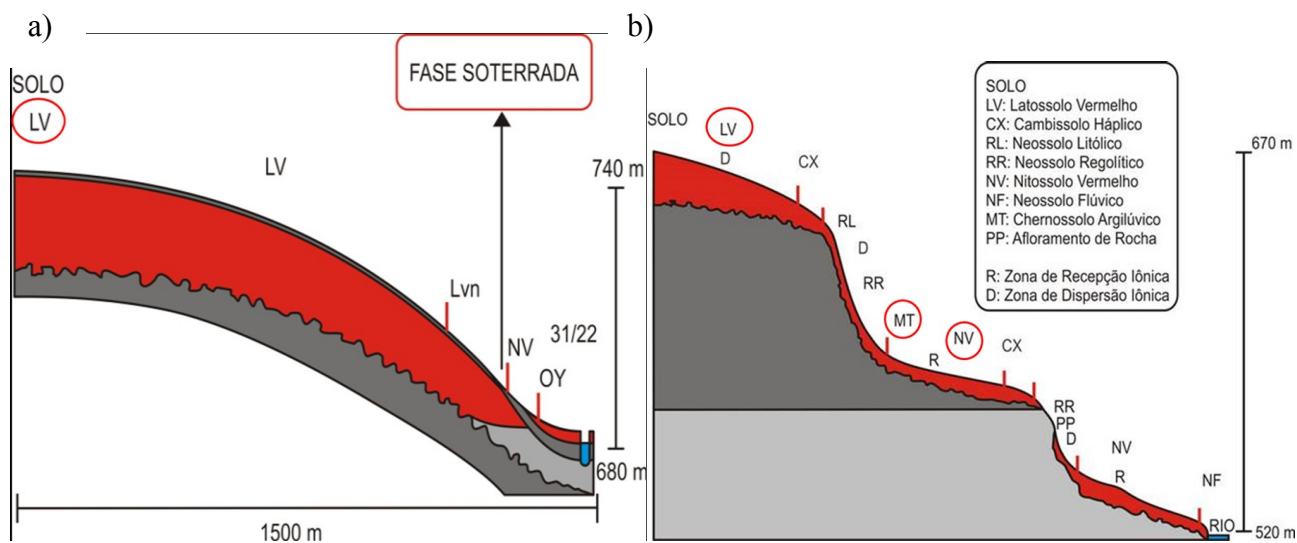
Figura 4.1. Representação esquemática da pedossequência a) convexada e b) patamarizada da Formação Serra Geral. Adaptado de Curcio (2006).
