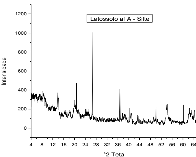
Apêndice 1. Difratoigramas de raio-X das frações granulométricas dos horizontes estudados.
