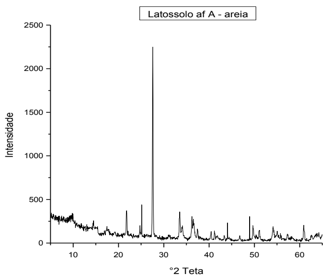
Apêndice 1. Difratoigramas de raio-X das frações granulométricas dos horizontes estudados.
